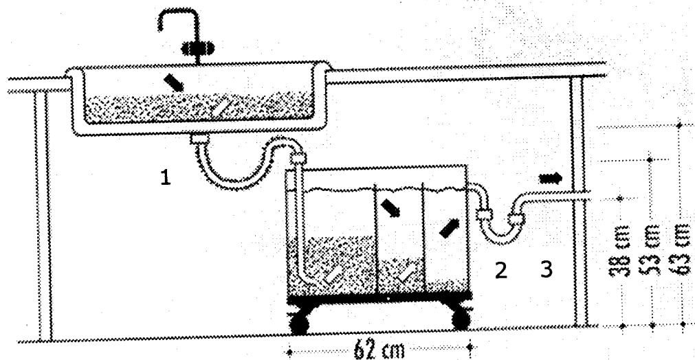
Schematische opstelling van de kleislib separatiecontainer Deze kan per situatie verschillend zijn.
